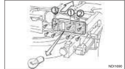
Hintere Kombinationsleuchte (Richtungsblinker/Bremsleuchte/Rückfahrleuchte) (Modelle ohne Ladefläche)
