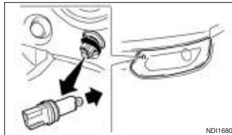
Begrenzungsleuchte (Glühlampen-Typ)
