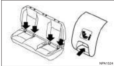
Lage der i-Size-ISOFIX-Ankerpunkte
