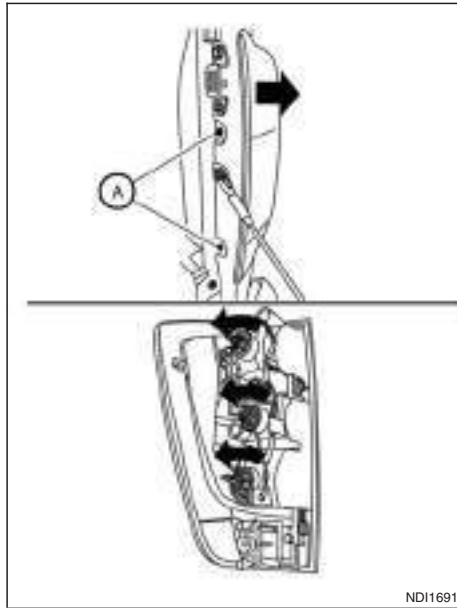
Hintere Kombinationsleuchte (Richtungsblinker/Bremsleuchte/Rückfahrleuchte) (Modelle mit Ladefläche)
