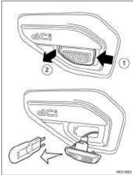
Seitlicher Richtungsblinker (an der Frontschürze) (falls vorhanden)
