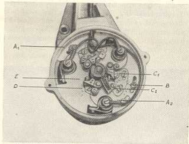
Bild M 52. Grundplatte des Dreihelunterbrechers um die Kontakthebelschnecke etwas geschwenkt und dadurch der Abstand verkleinert oder vergrößert werden kann. Nach dem Wiederfestziehen der Schraube D ist der Kontaktabstand nochmals zu überprüfen. Anschließend an jedes Nach- oder Neueinstellen der Zündung sind auch die Kontaktabstände nachzuprüfen.
