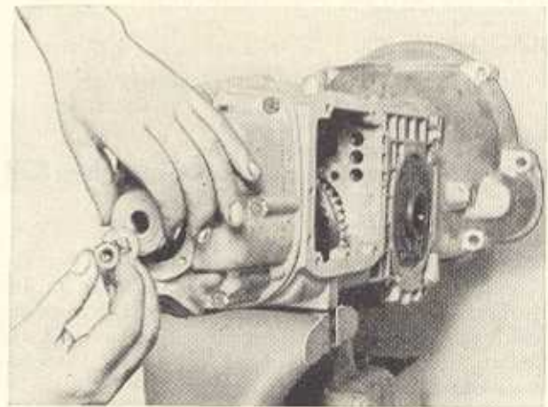
Bild G 84. Aufsetzen des Tachoantriebsrades
