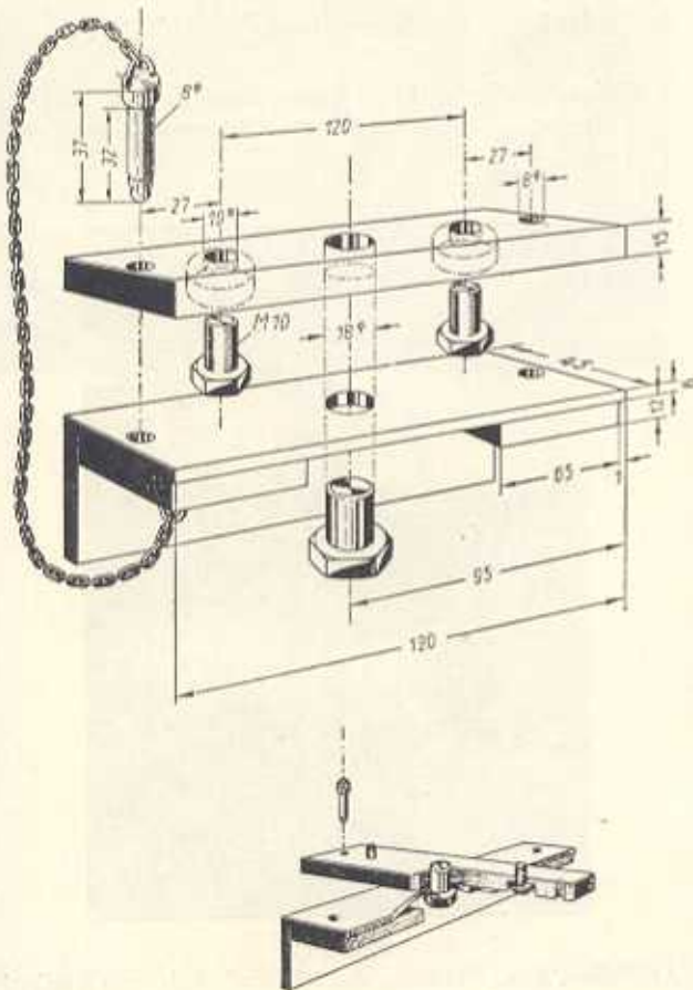
Bild G 11. Maßskizze der Haltevorrichtung für Getriebe
