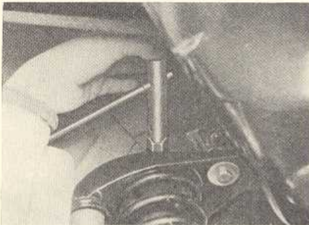
Bild F 65. Lösen des oberen Stoßdämpferanschlusses beim Baumuster 312
