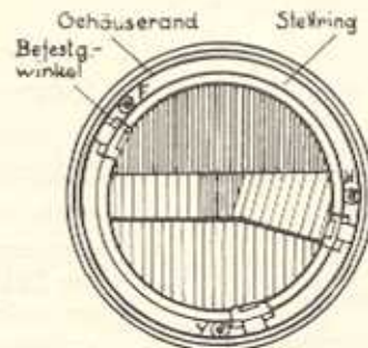
Bild E 4. Einstellschrauben am Scheinwerfer
