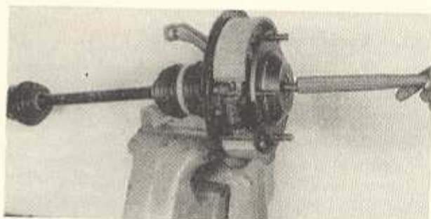
Bild F 36. Herausdrücken der Gelenkwelle aus dem Radantrieb
