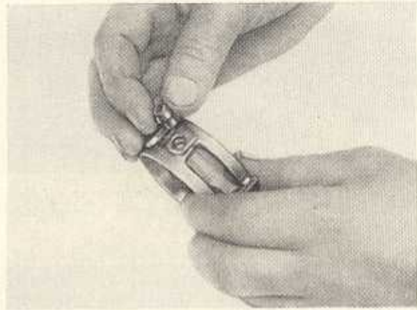
Bild G 57. Einsetzen der Sperrstifte in den Synchronkörper
