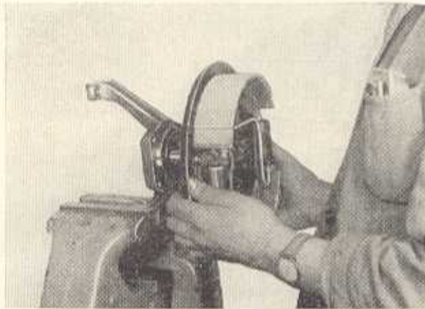
Bild F 47 Aufstecken der Vorderradbremse auf das Billenlager 6307
