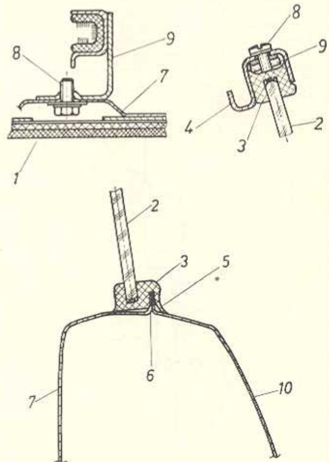
Bild K 34. Seitenscheibe der Hintertür
