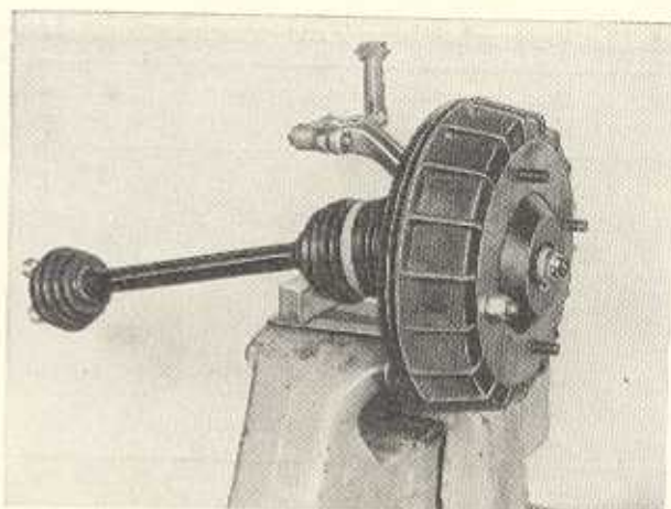
Bild F 35. Vorderradantrieb im Schraubstock mit Weichmetallbacken eingespannt
