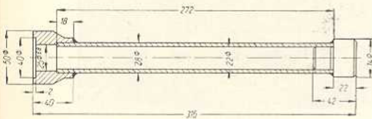
Bild G 63. Maßskizze für Hobdorn W-86 922/1
