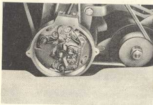
Bild M 48. Zur Wartung am Fahrzeug vorbereiteter Anbau-Dreihelunterbrecher beim Baumuster 312
