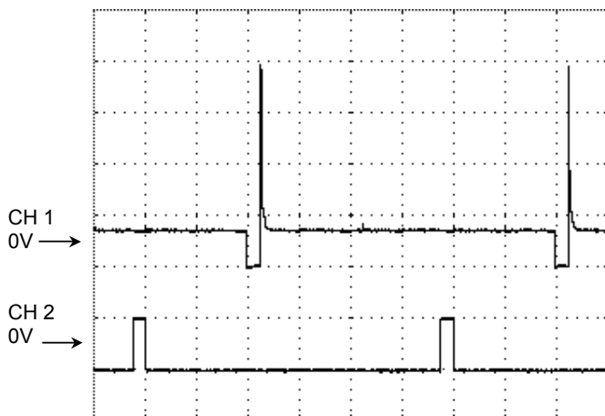
Forma de onda de referencia de la señal de control del inyector y bobina de ignición
