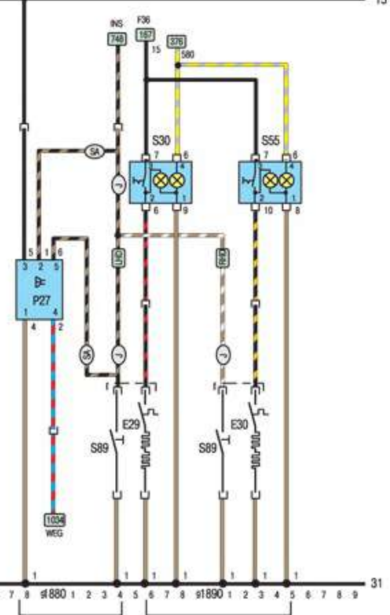
СИГНАЛИЗАЦИЯ
