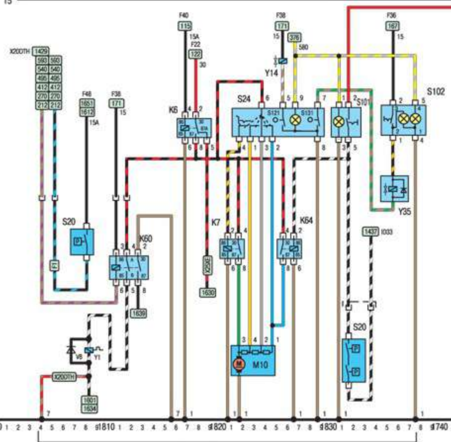
КОНДИЦИОНЕР
