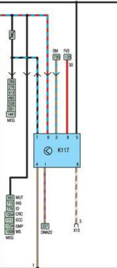
ИММОБИЛИЗАТОР
