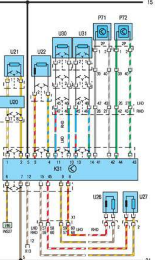
ПОДУШКА БЕЗОПАСНОСТИ
