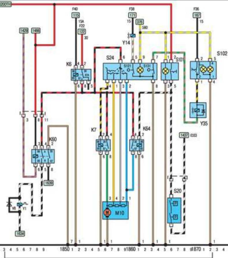
КОНДИЦИОНЕР
