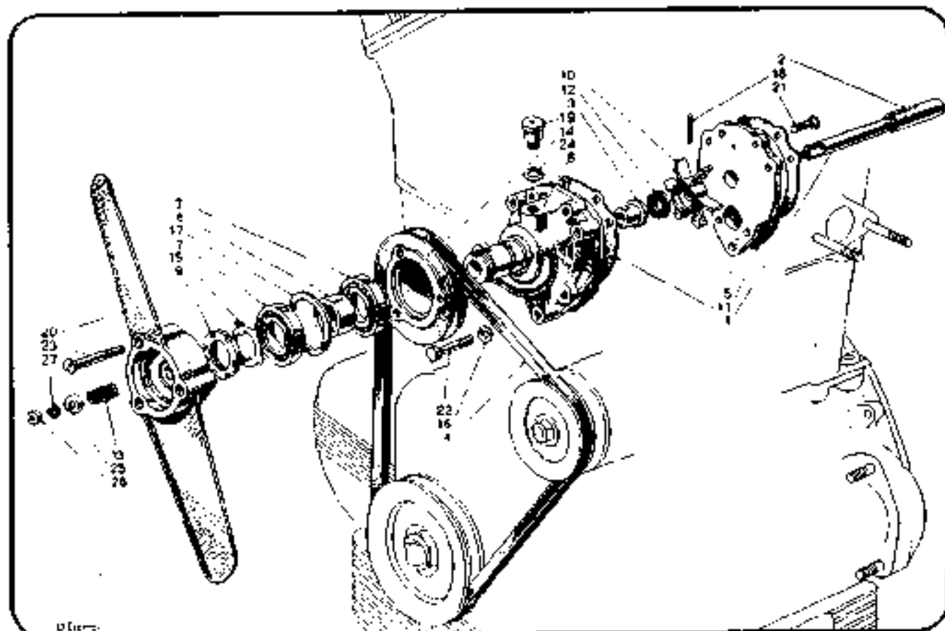
Fig. 01/28 - Pompa acqua - Ventilatore motore 1ª serie (Da' Catalogo parti di ricambio).
