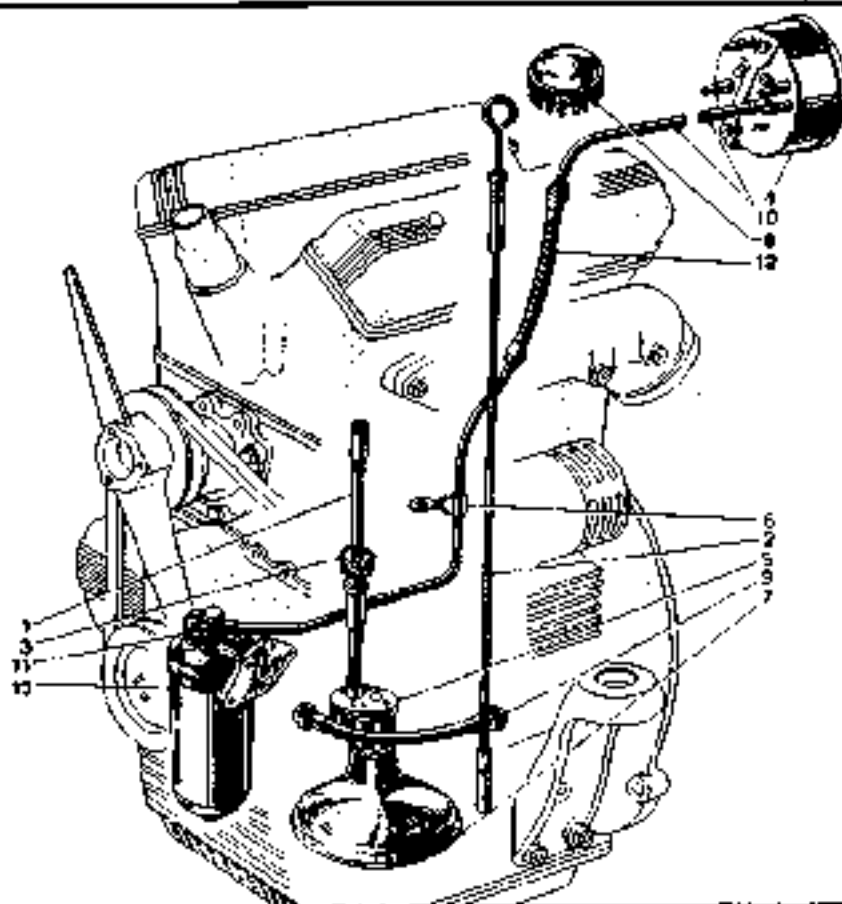
Fig. 00/2 - Schema della lubrificazione (Dal catalogo parti di ricambio).
