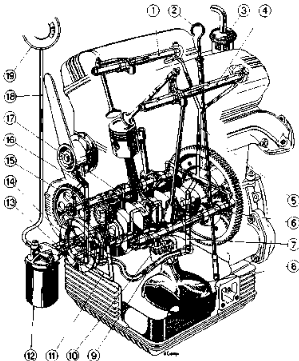
Fig. 01/27 - Lubrificazione motore
