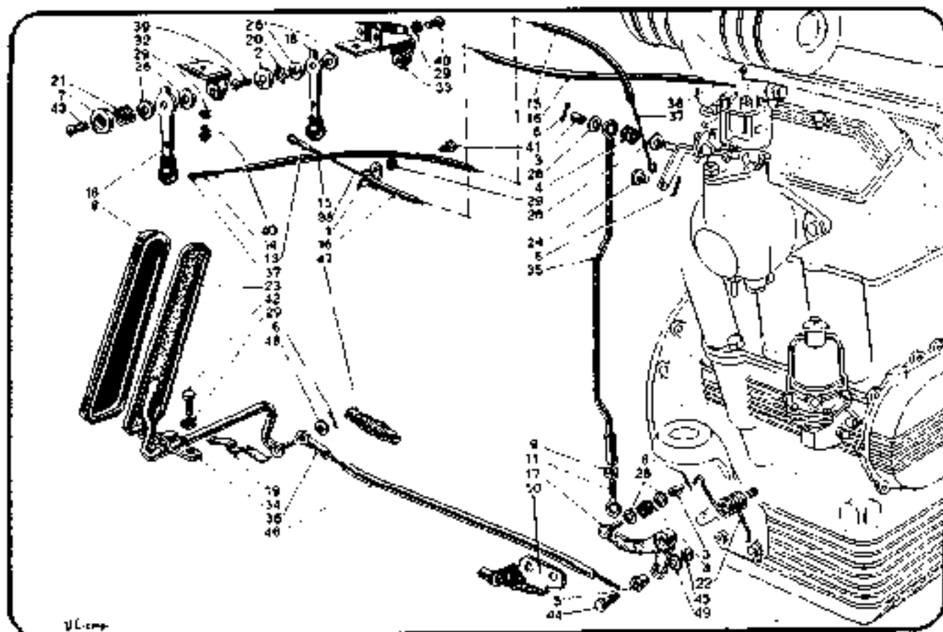
Fig. 01/18 - Comando a ruota ed a pedale acceleratore. Comando articolato (Dal Catalogo parti di ricambio)
