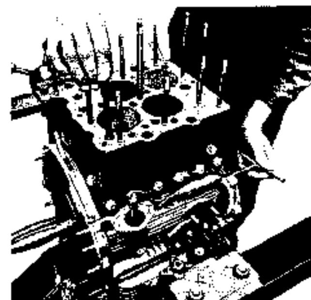
Fig. 01/21 - Posizione dell'alberino del distributore d'accensione.
