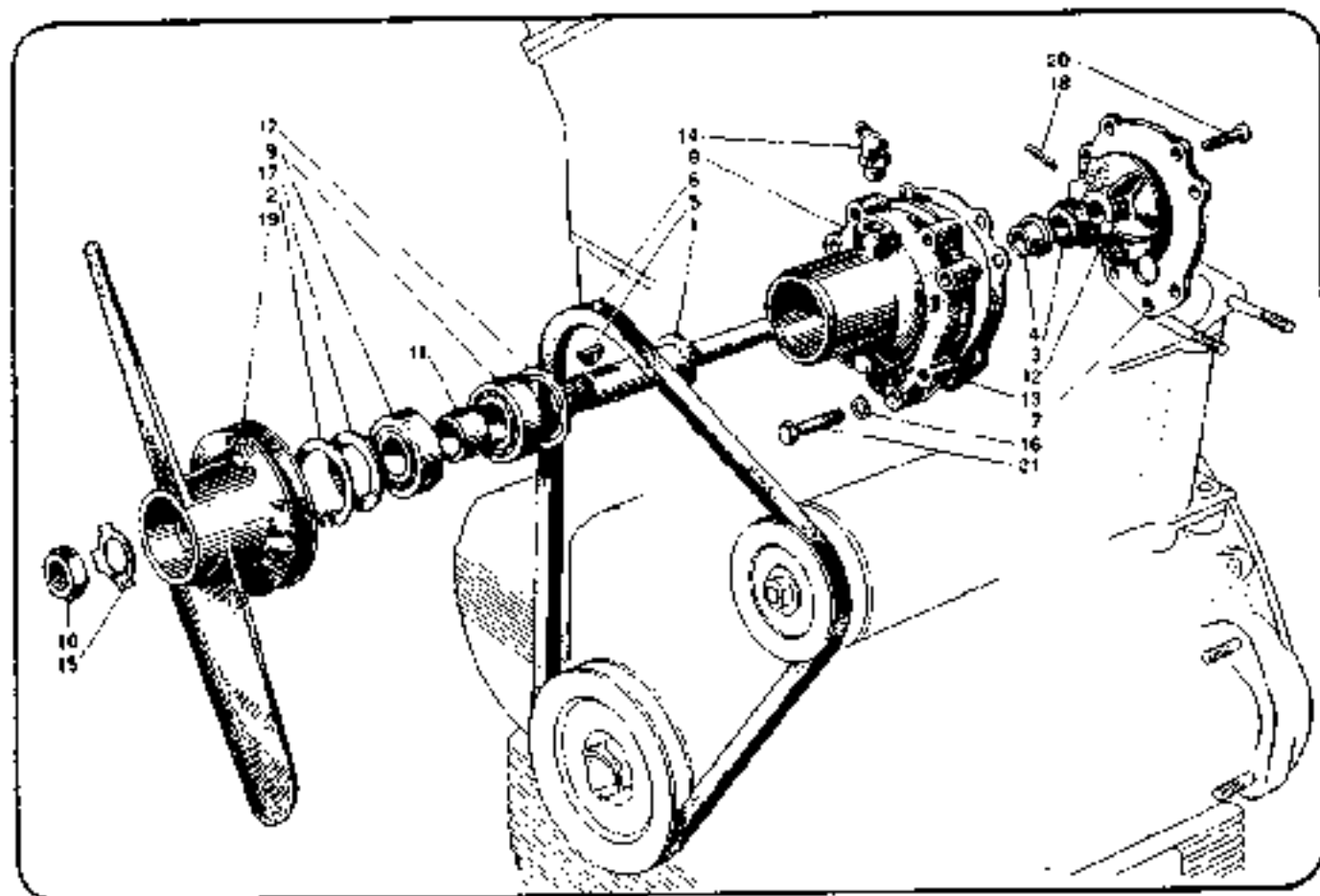
Fig. 81/34 - Pompa acqua - Ventilatore motori 2° e 3° serie (Del Caricatore parti di ricambio)
