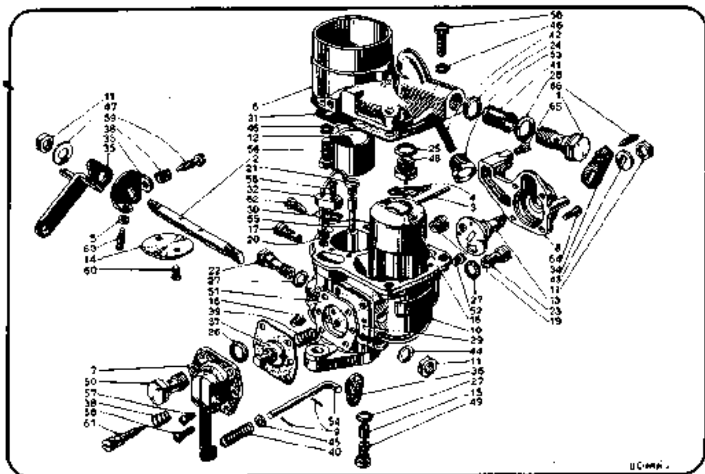
Fig. 01/25 - Carburatore per motori 2° e 3° serie (Del Coloforo parti di ricambio)
