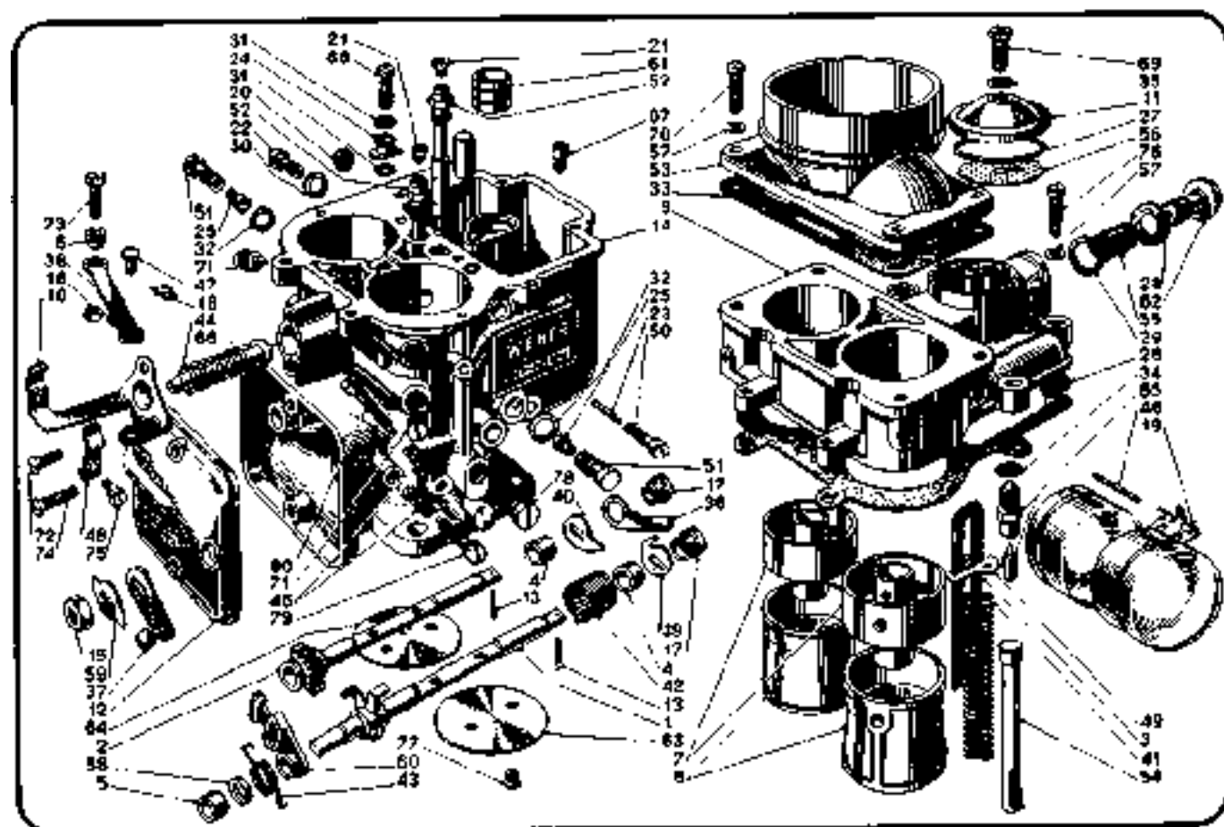
Fig. 01/31 - Carburatore per motori catalani (Da) Catalogo parti di ricambio.
