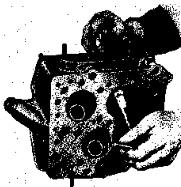
Fig. 01/26 - Ripassare alloggiamento sedi valvole.
