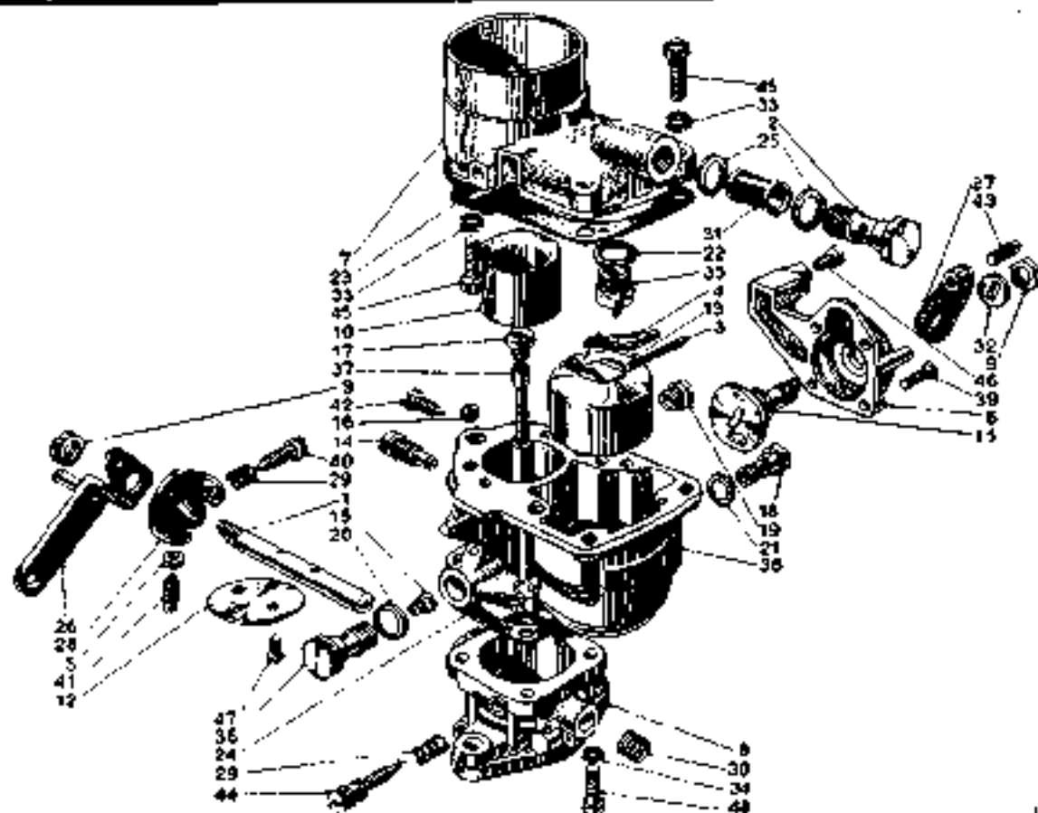
Fig. 01/29 - Carburatore motore 1° serie (Dal Catalogo parti di ricambio).
